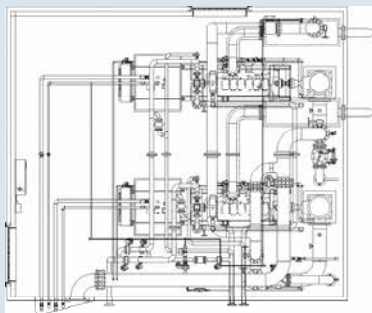
Prefab pompkamer
